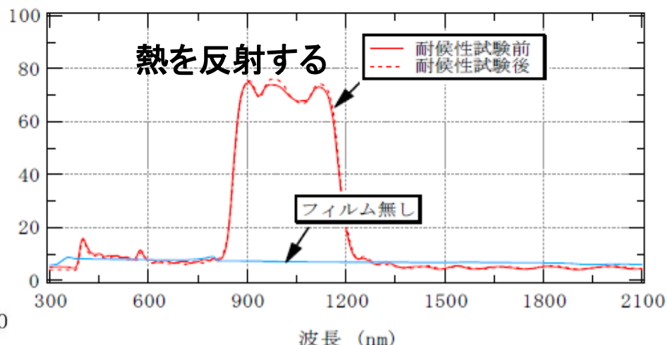
分光反射率 (%)
