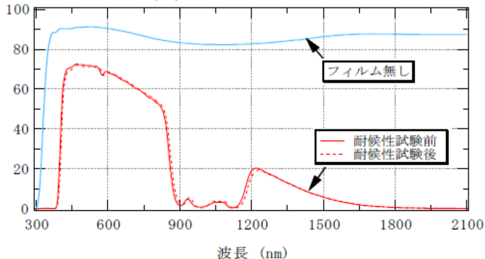
分光反射率 (%)
