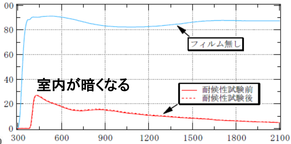
分光透過率 (%)
