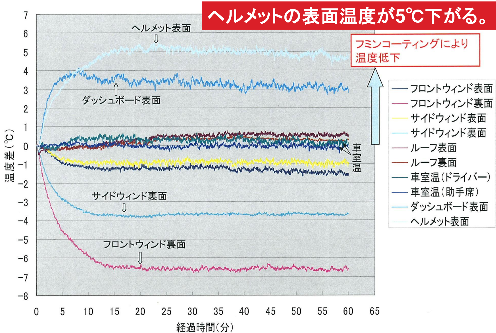
図1. 各部温度差(ノーマル - フミン)
